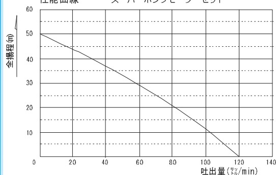
性能曲線 スーパーポンプモーターセット
