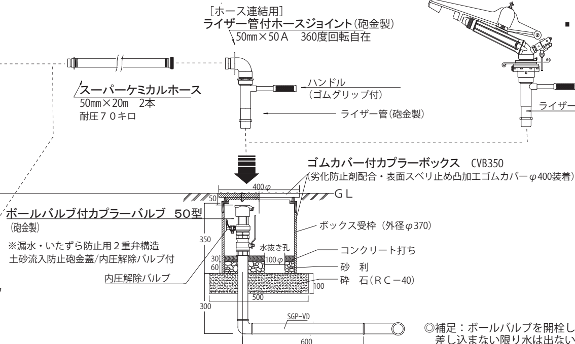
ライザー管付ペロットスプレーガン 50.R-ZN
