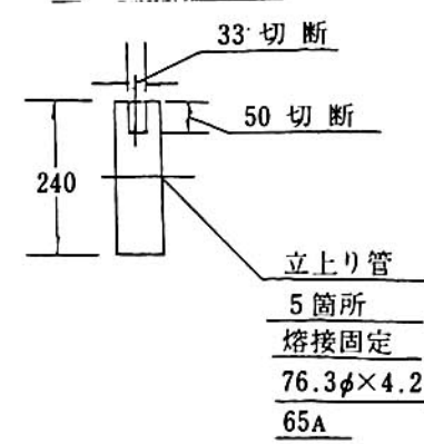
② 立面図
