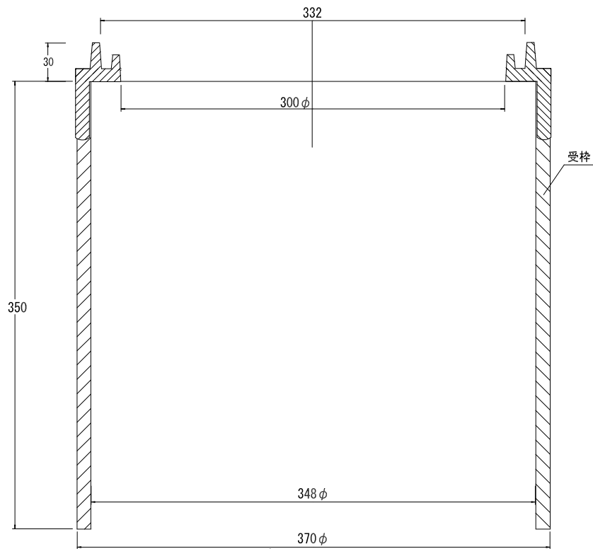
ケーブルボックス枠
