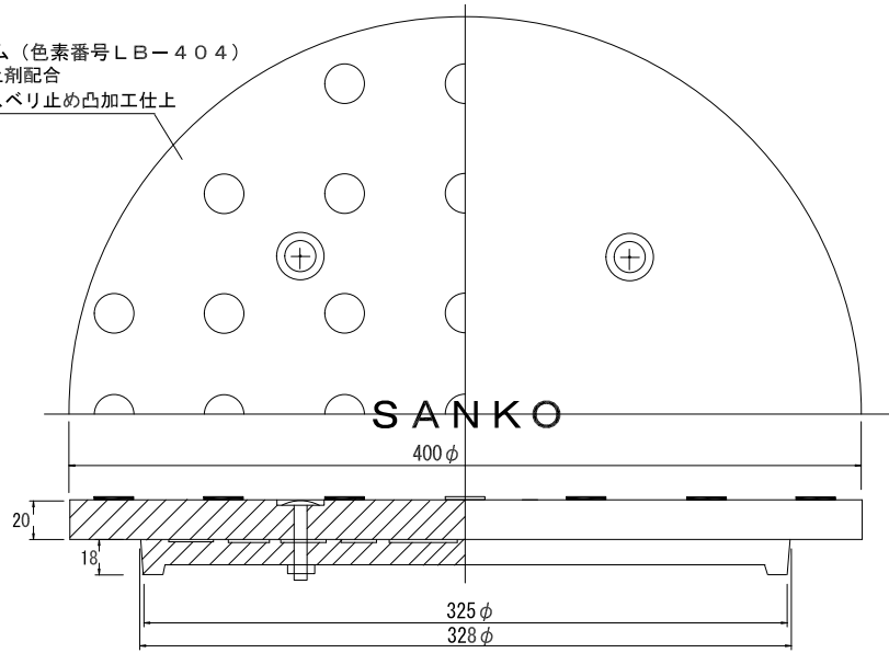
ケーブルボックス蓋 (緑色ゴムカバー付)
