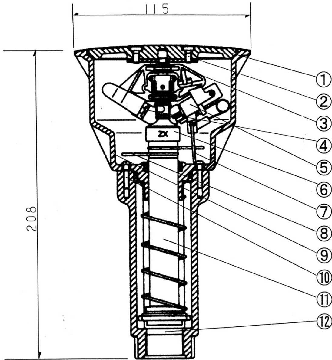
取付口径 20 mm (メスジ)
