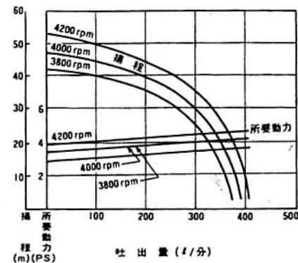
性能曲線図
