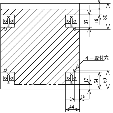
ボックス取付穴推奨寸法ト背面加工スペース
