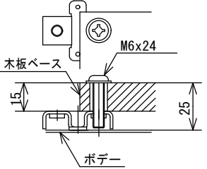
ベース取付部詳細 (1/2)
