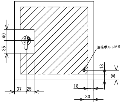
扉機器取付有効図
