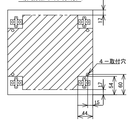
ボックス取付穴推奨寸法ト 背面加工スペース
