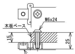
ベース取付部詳細 (1/2)
