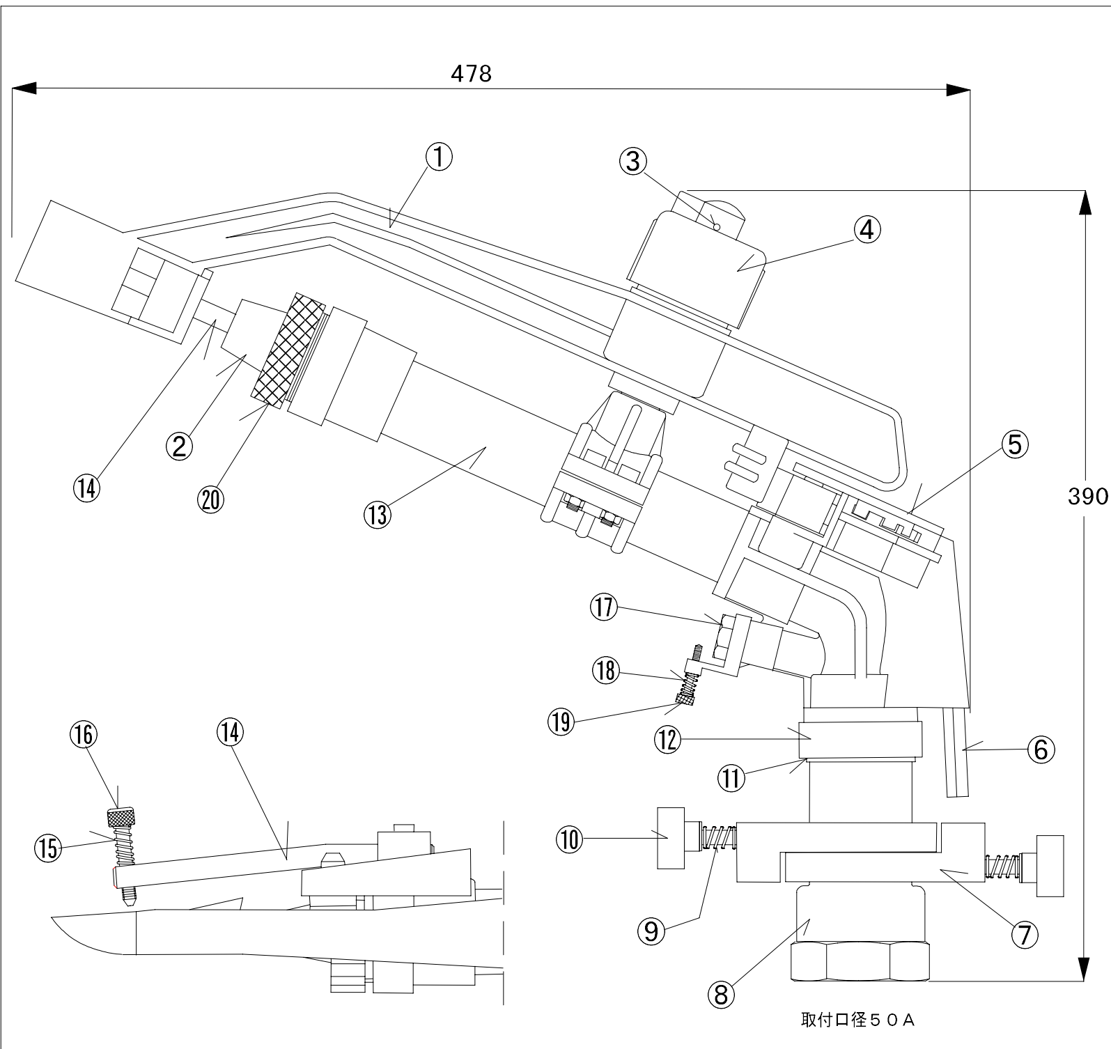
図名 スプレーガン SG1-T (2ノズル)
